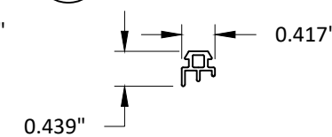
15 HEAD GASKET EPDM
