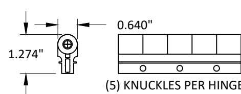
23 CENTER HINGE ALUMINUM 6063-T5
